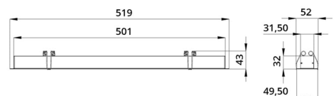
Габаритный чертеж
