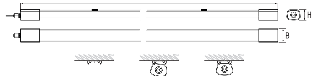
Рис.1 Схема монтажа светильника PWP-C4
