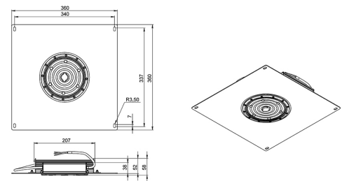
Монтаж светильника
