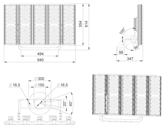
Габаритный чертеж
