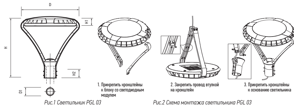
Рис.1 Светильник PGL 03
